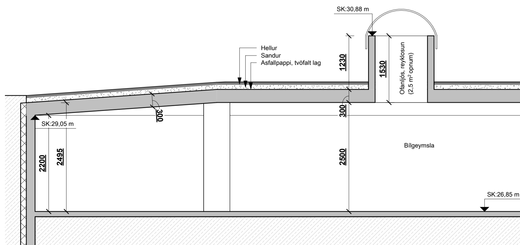
SNÍÐ D-D mkv: 1 : 50
