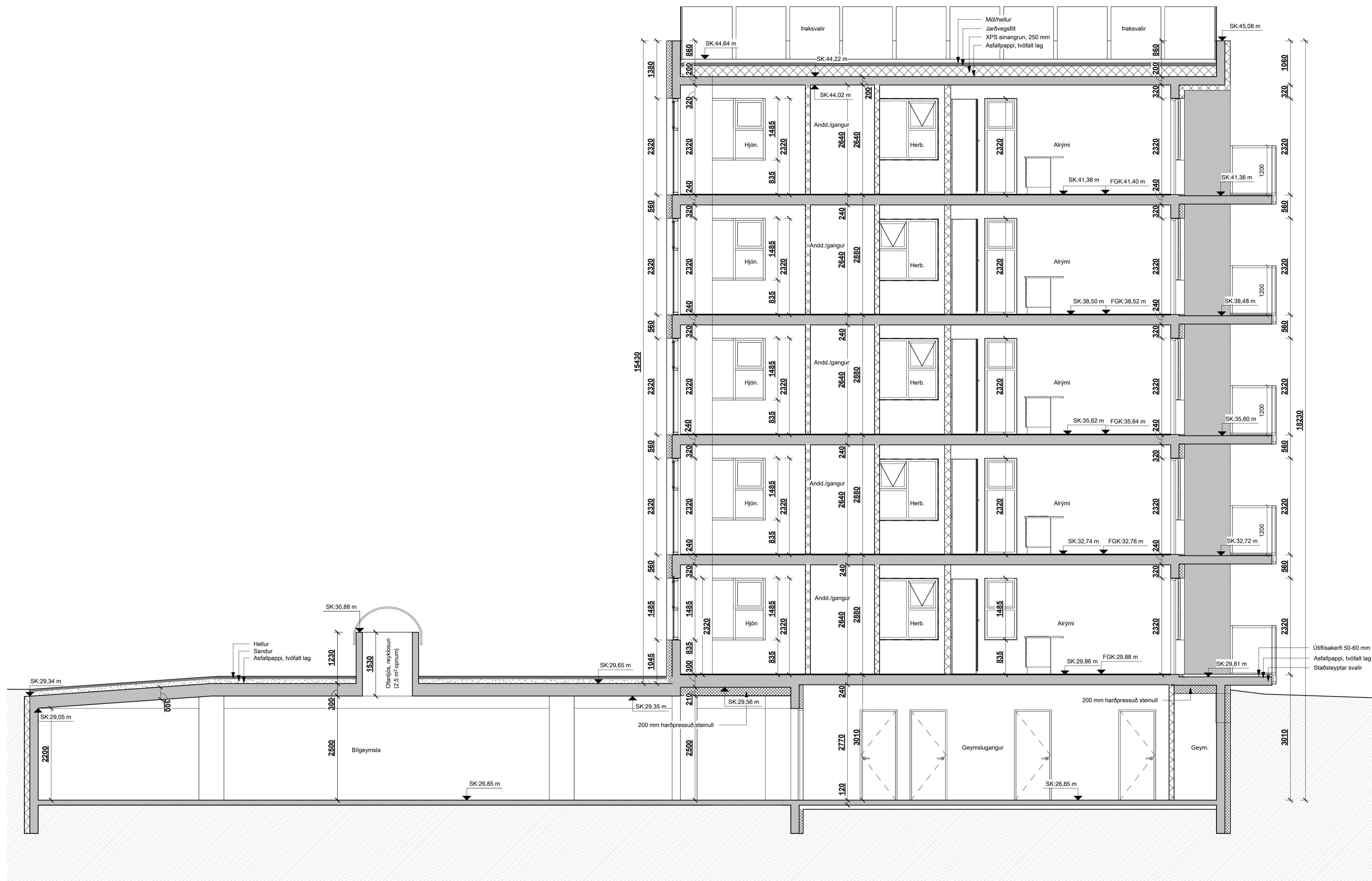
SNID E-E mkv: 1 : 50
